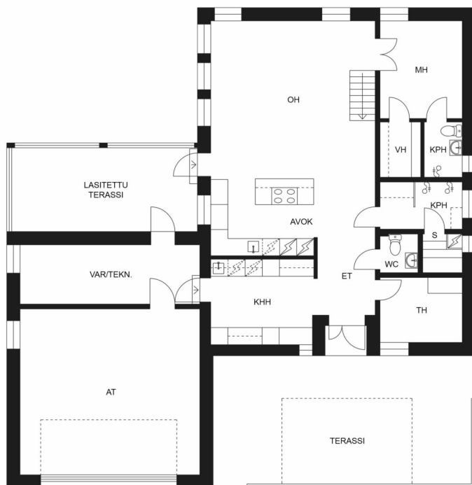
1.KERROS
