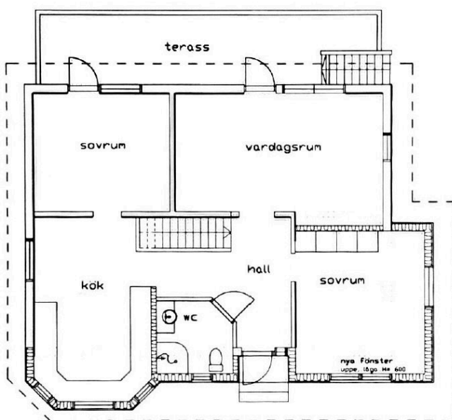
övre Plan
