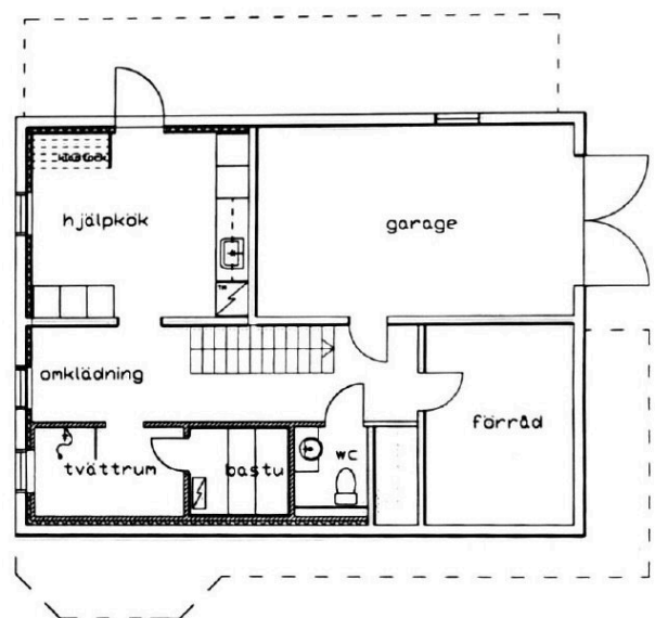
Källarplan
