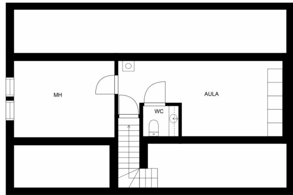
2. KERROS
